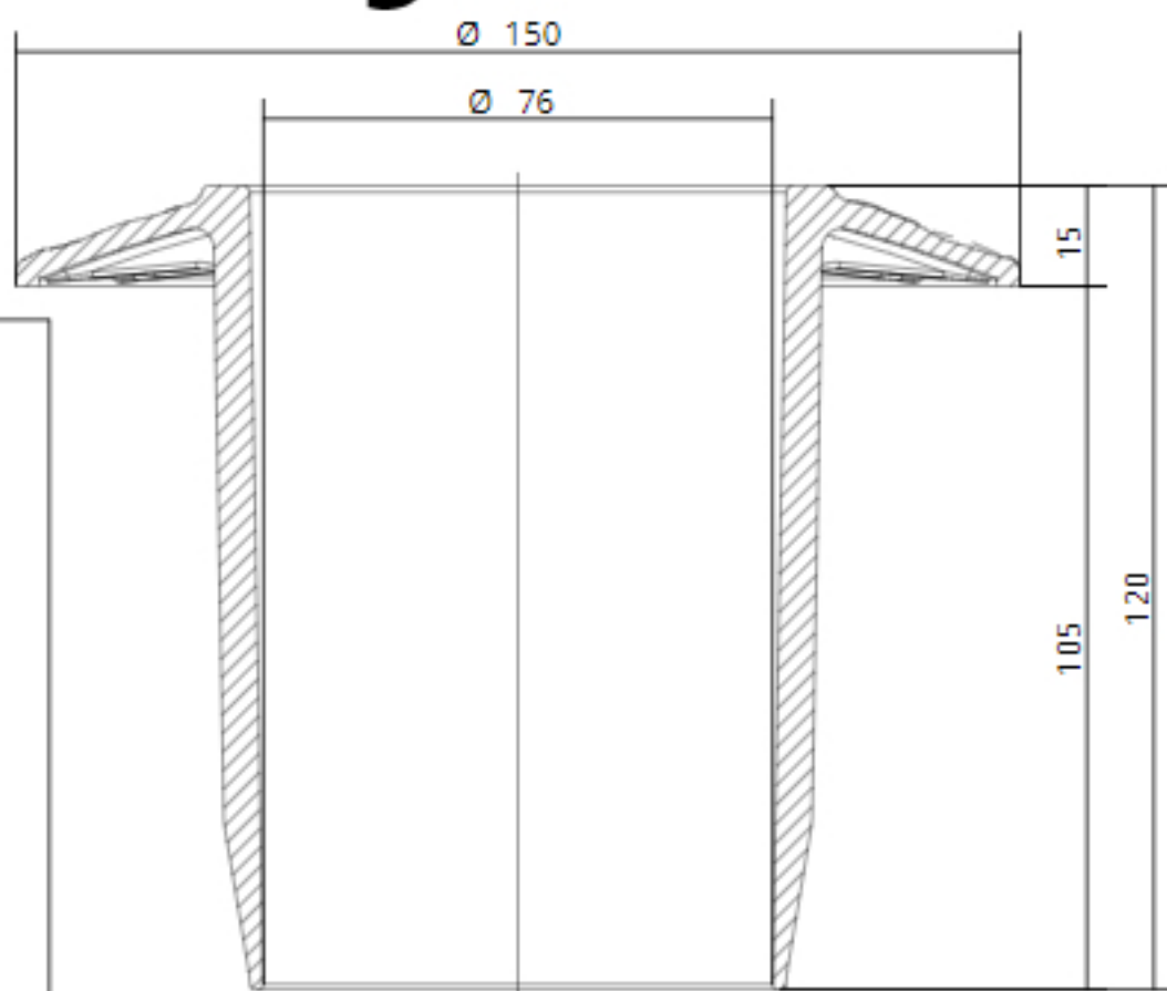
Sez. A-A
