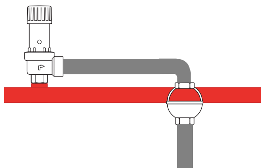
Fig.1 Installazione diretta dell'imbuto sulla tubazione di scarico
