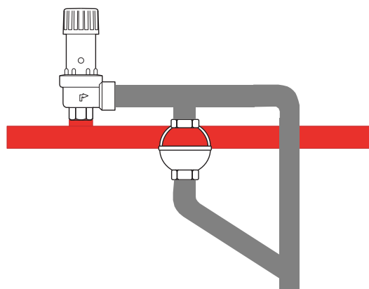
Fig.2 Installazione tipica dell'imbuto in presenza di alta portata di scarico
