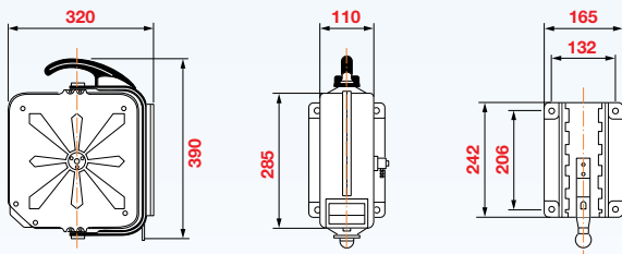
DIMENSIONI D'INGOMBRO
